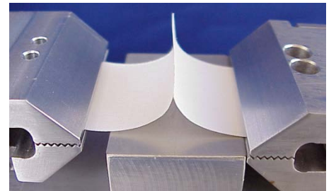
90° peel
