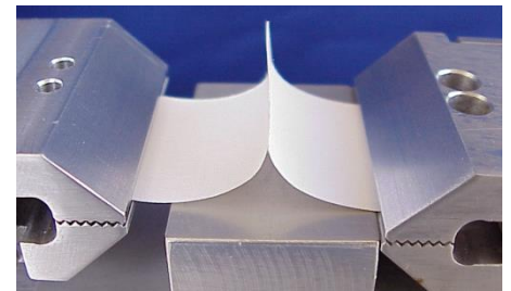
90° peel
